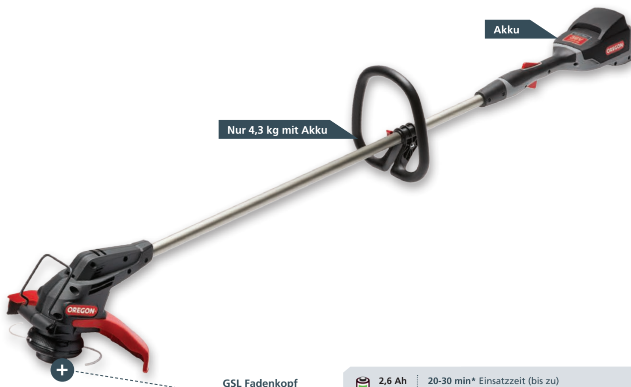
GSL Fadenkopf
